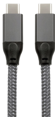
USB 3.2 Gen 2x2 Kabel, USB-C - USB-C, 20 Gbit/s, 5A, 100W
